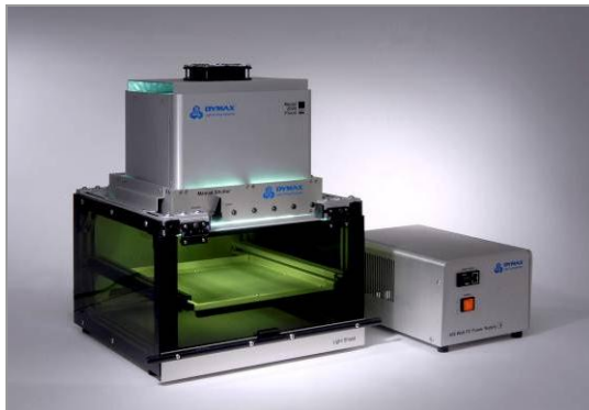
Dymax 2000-PC Flächenstrahler mit Blende und Abschirmung. Mittlere Intensitäten für die Aushärtung einzelner Bauteile oder von mehreren Bauteilen gleichzeitig. Bestrahlte Fläche von 200 x 200 mm.
