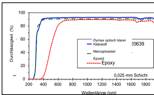
Dymax Klebstoffe der OP-Serie zeichnen sich durch sehr gute optische Transmission aus
