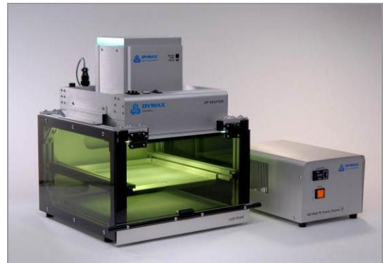
Dymax 5000-PC Flächenstrahler mit Blende und Abschirmung. Mittlere bis hohe Intensitäten für die Aushärtung einzelner Bauteile oder von mehreren Bauteilen gleichzeitig. Bestrahlte Fläche von 120 x 120 mm.
