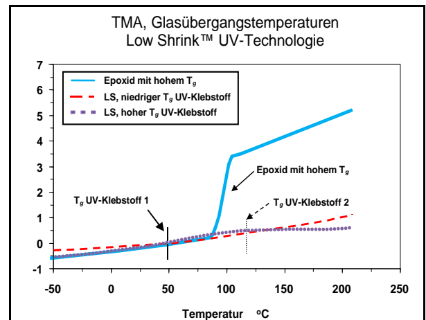
Dauerhafte Verklebung durch eine minimale Relativbewegung zwischen den Füge-teilen bei Temperaturänderungen
