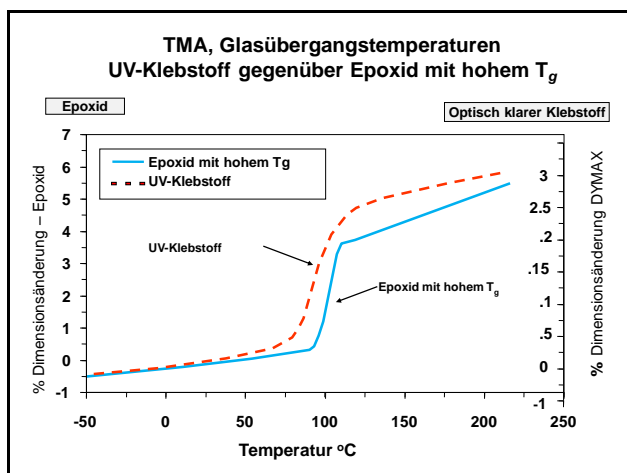
Hohe T g -Werte neuartiger UV-Klebstoffe im Vergleich zu Epoxiden
