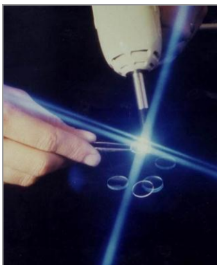
Linsenverklebung
